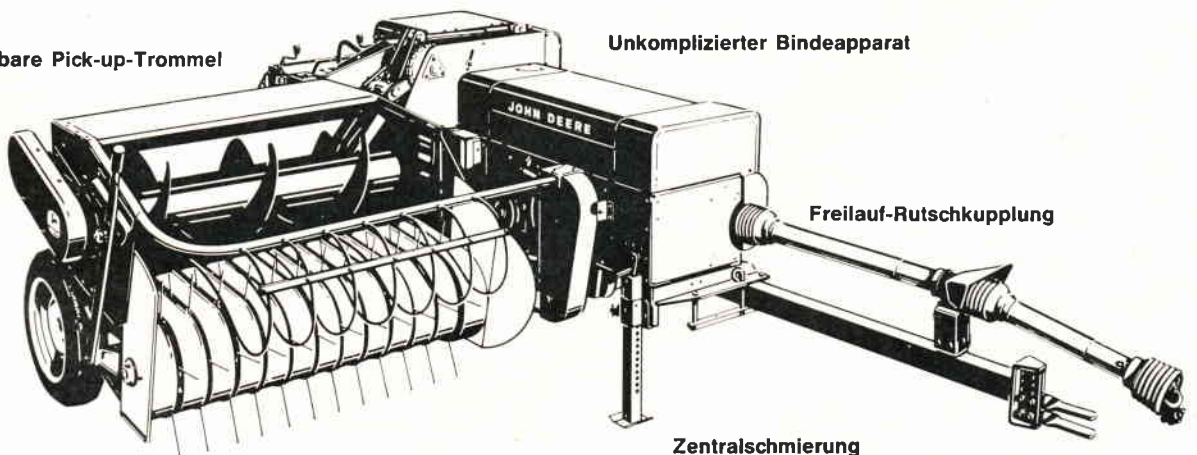
Zentralschmierung
